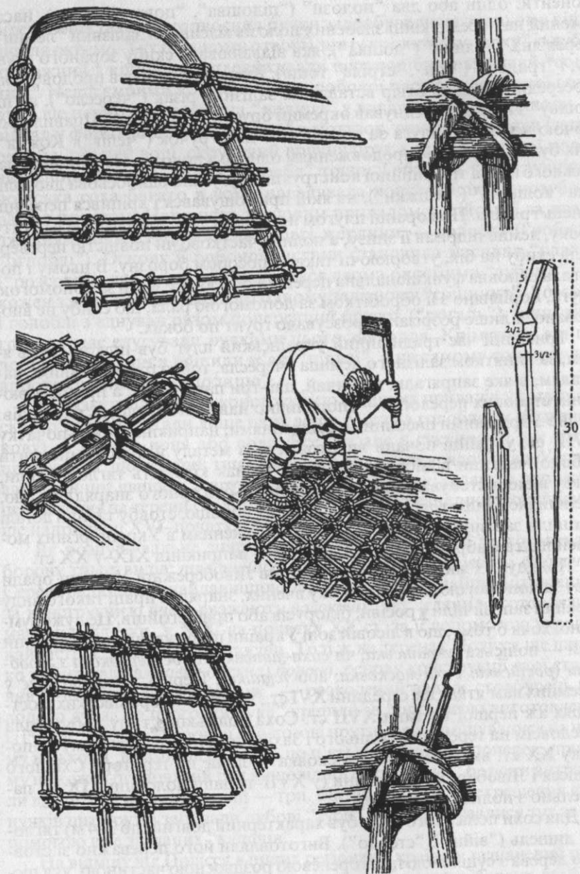
Технологія складання польської борони
