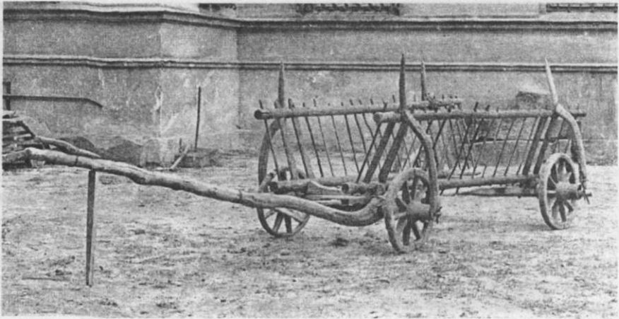
Воловий віз традиційної конструкції
